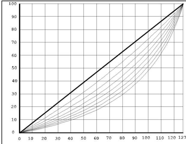
Fahrstufenkennlinie *)
