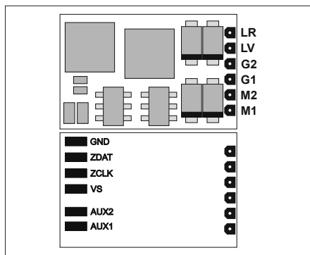
DH10C
