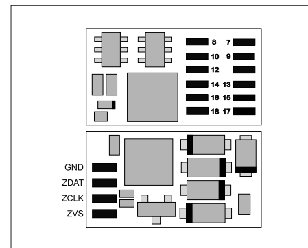
PluX12-Schnittstelle
