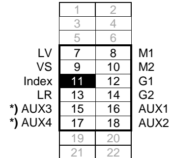
PluX12-Schnittstelle
