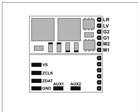
DH05C
