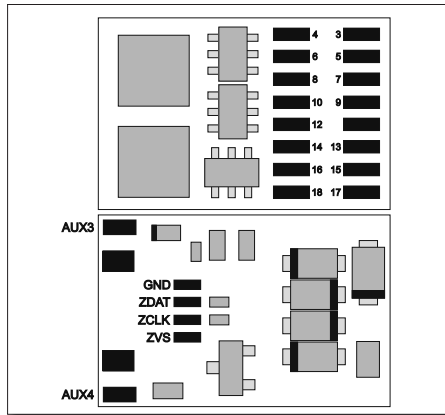
PluX16-Schnittstelle
